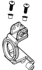
BS502-019 C Hub Unit(Rr)
